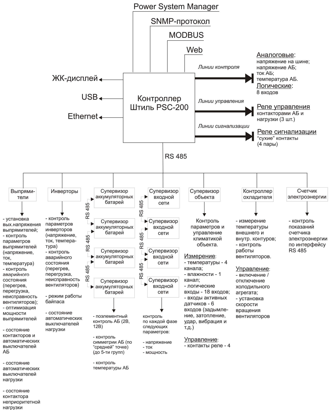
Рисунок 1. 4 - Структура контроллера Штиль PSC-200 (максимальная конфигурация)
